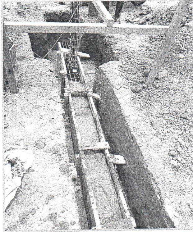
FOTO N°10: Colocación de Acero para Zapatas en Muro de Contención .
