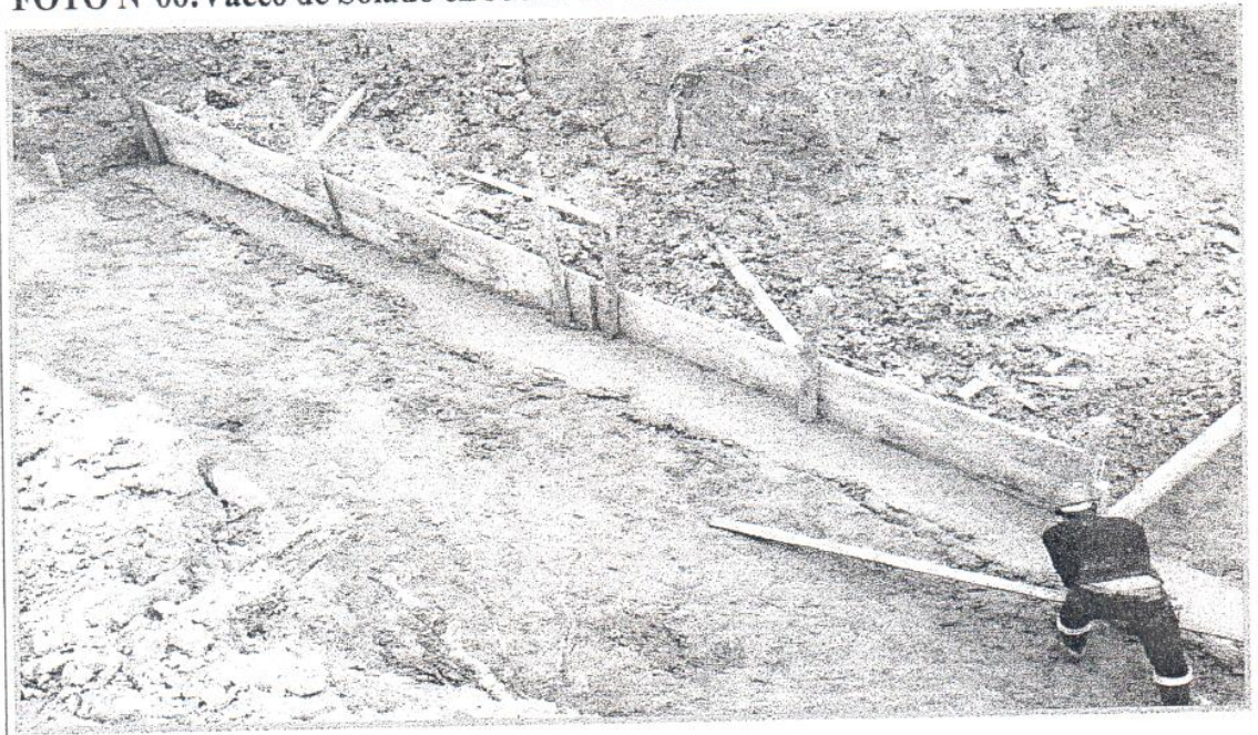
FOTO N°06: Vaceo de Solado en Muro de Contención.
