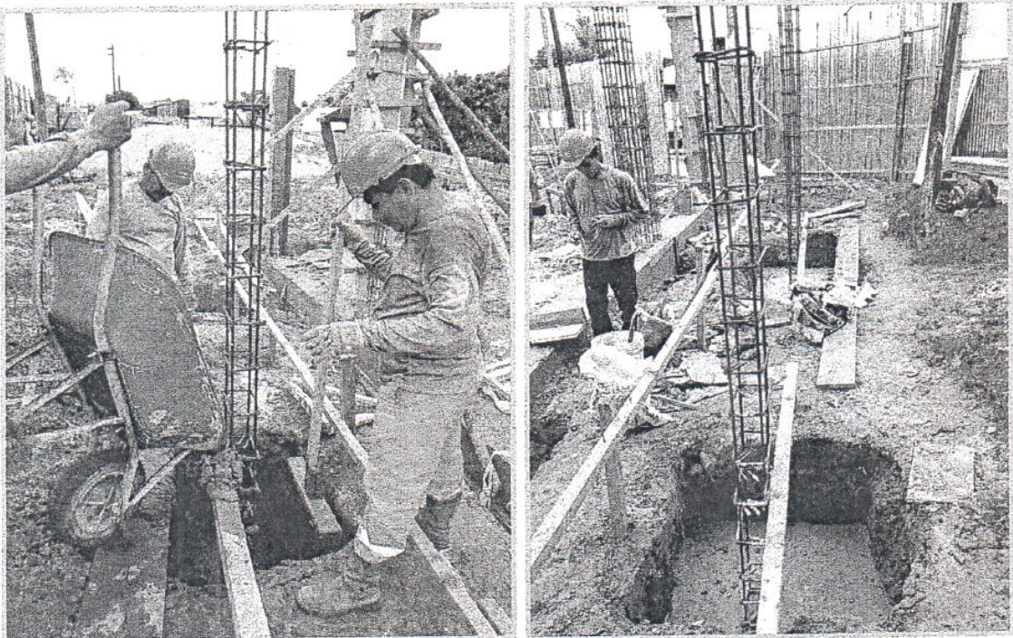
FOTO N°08: Vaceo de Mortero en Zapatas.
