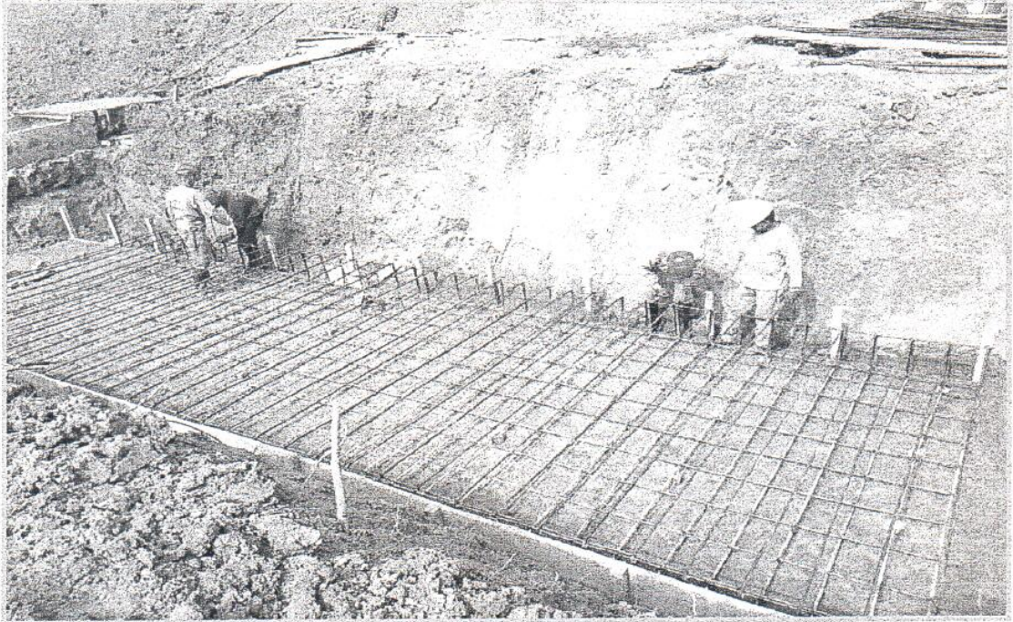
FOTO N°11: Colocación de Acero para Zapatas en Muro de Contención .
