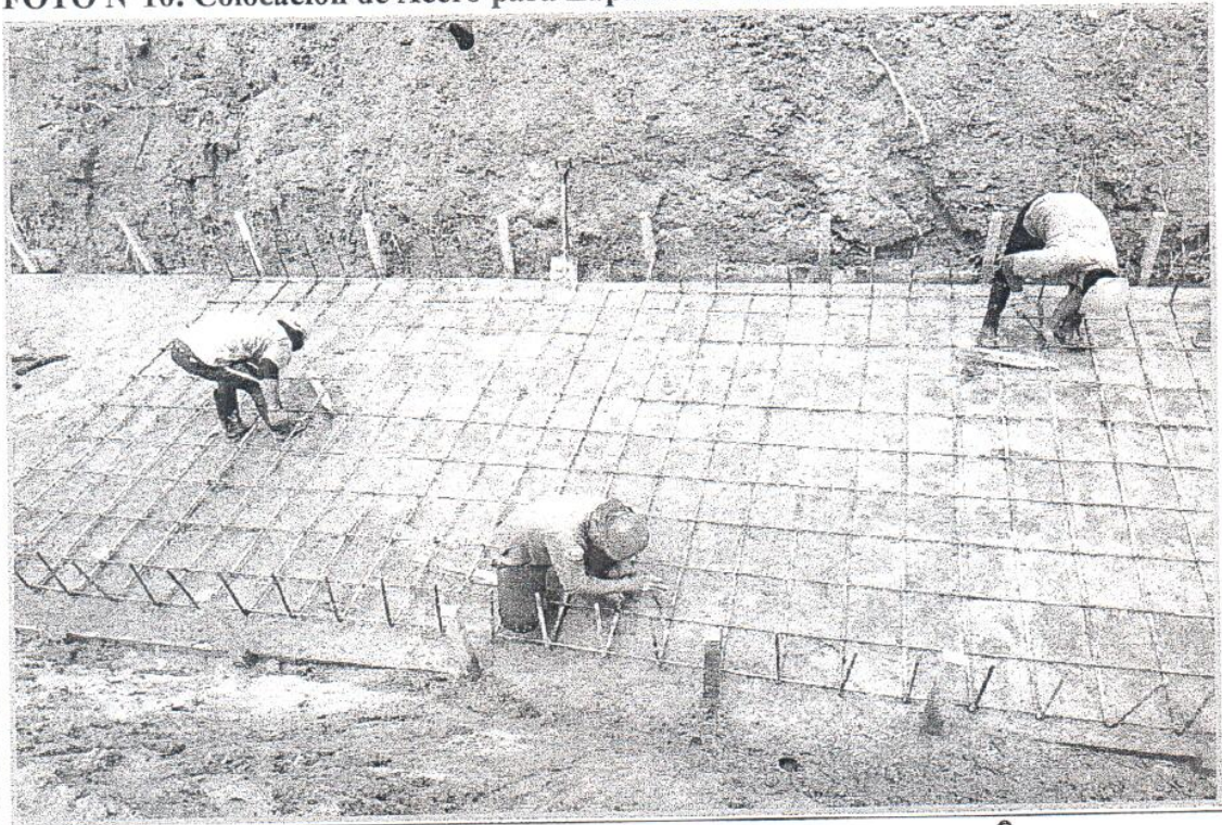
FOTO N°10: Colocación de Acero para Zapatas en Muro de Contención .
